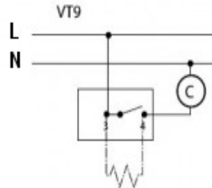
Thermostat sans position «arrêt» dégivrage par résistance
