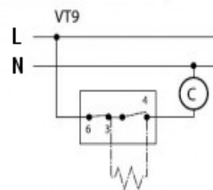
Thermostat avec position «arrêt» et dégivrage par résistance
